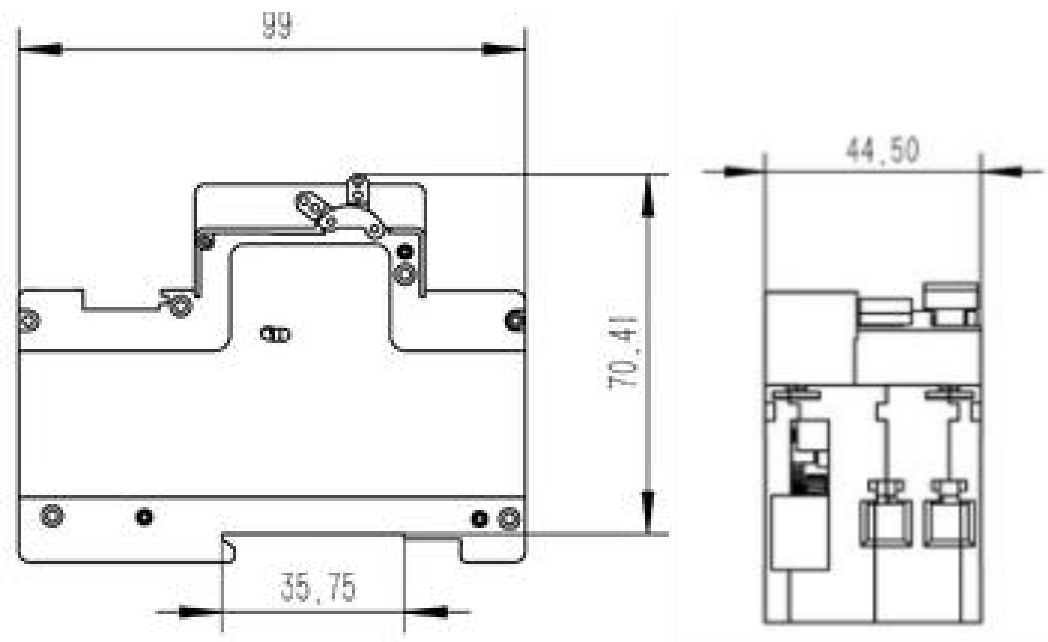
产品尺寸图
